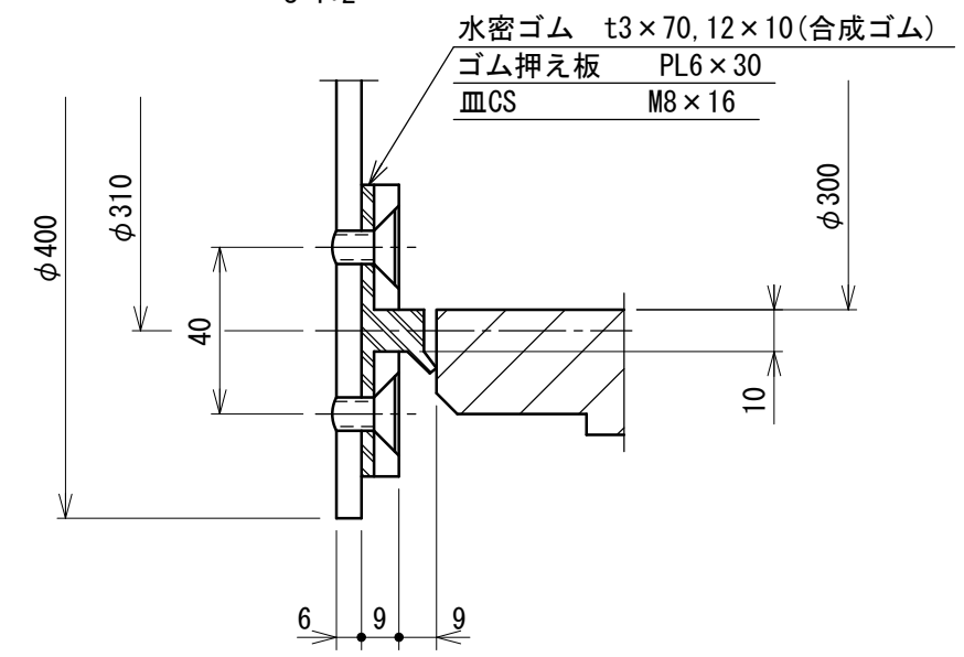
水密詳細
