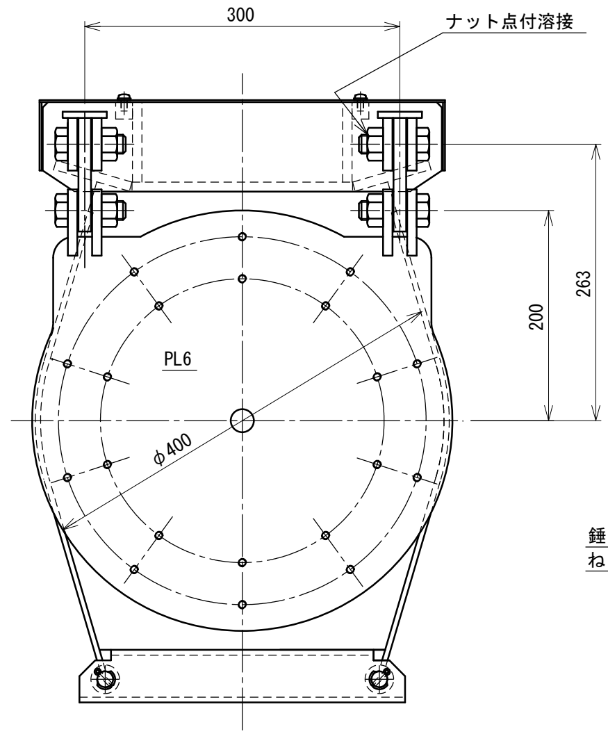
水密詳細
