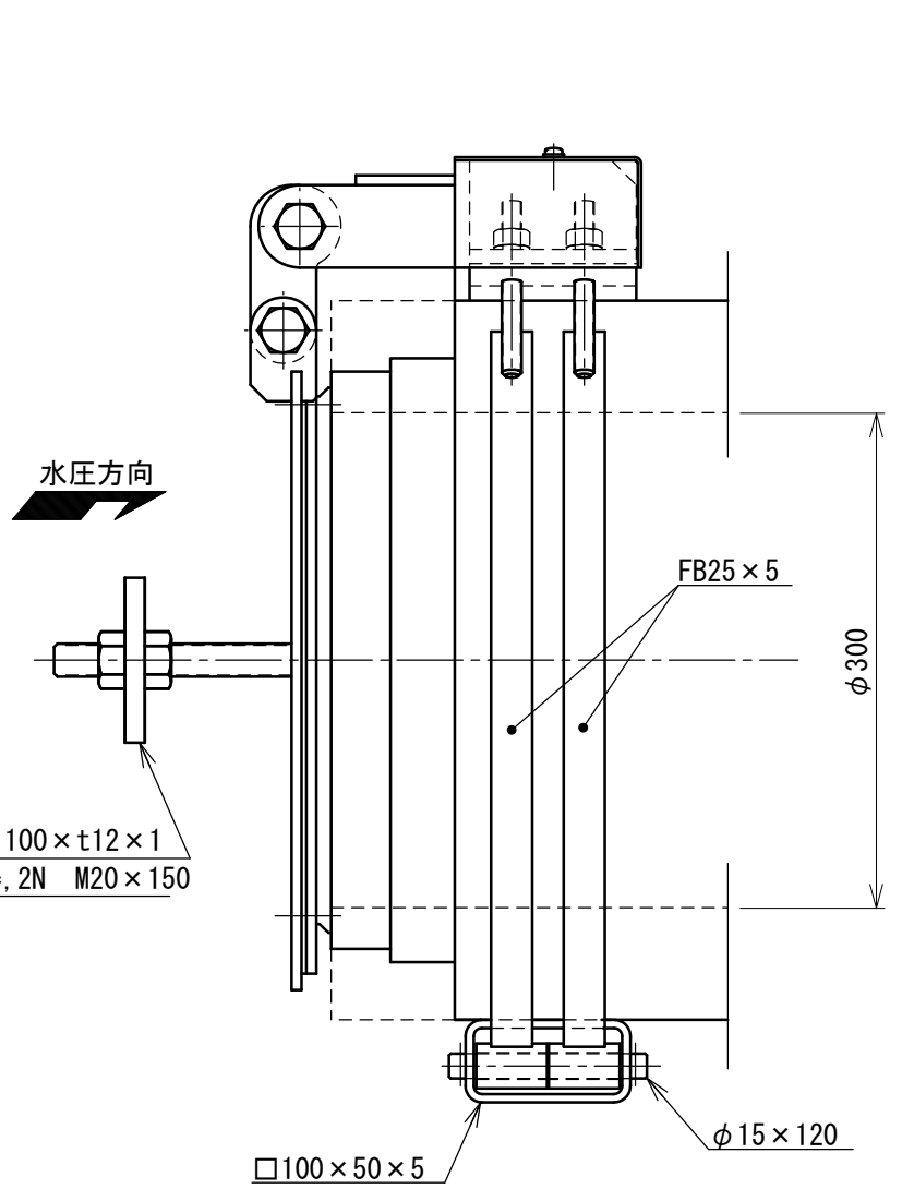
側面図
