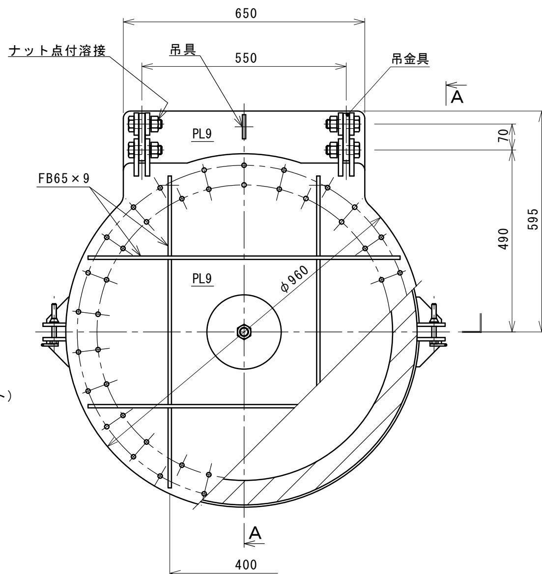
正面図 S=1:10
