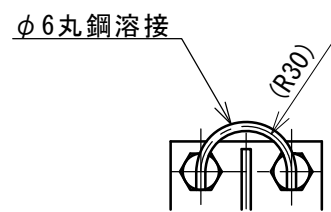
B-B S=1:5
